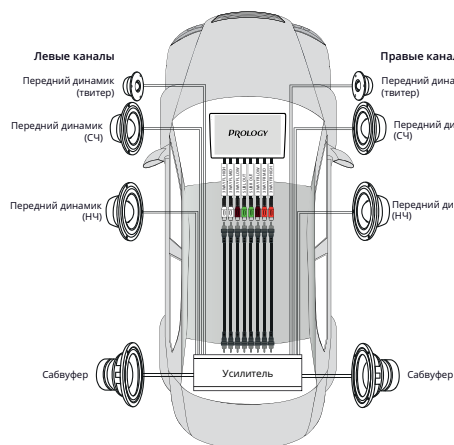
Подключение с использованием только RCA-выходов
